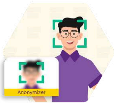
Face Anonymizer
